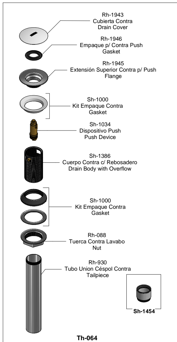
Th-064 Contra de Push para Lavabo sin Rebasadero Push Drain Lavatory without Overflow
