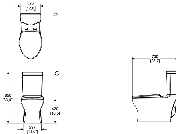
Medidas Referenciales / Estimated Dimensions, Acot. mm [pulg.] / Dim. mm [inch.]
